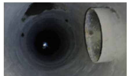
Nachher: Schacht komplett wiederhergestellt und vollumständig strukturell mit QLS GeoKrete.
